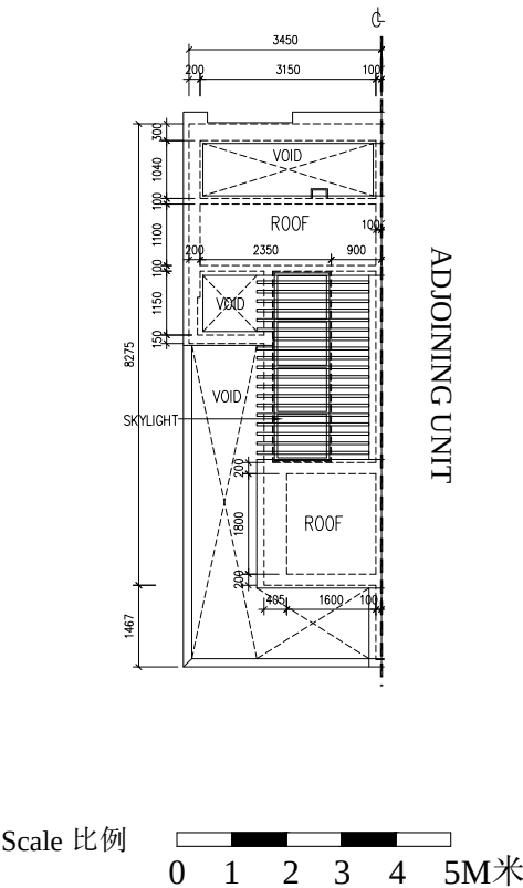
上層天台平面圖 Upper Roof Floor Plan
